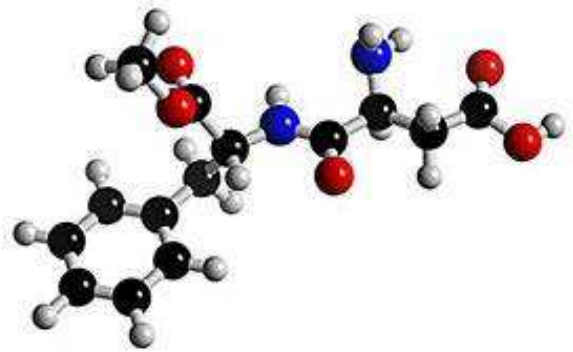
Aspartam Strukturmodell
