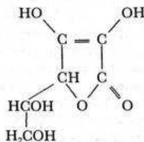
Ascorbinsäure
