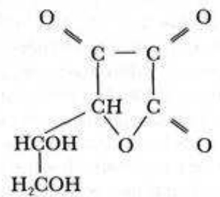
Dehydroascorbinsäure
